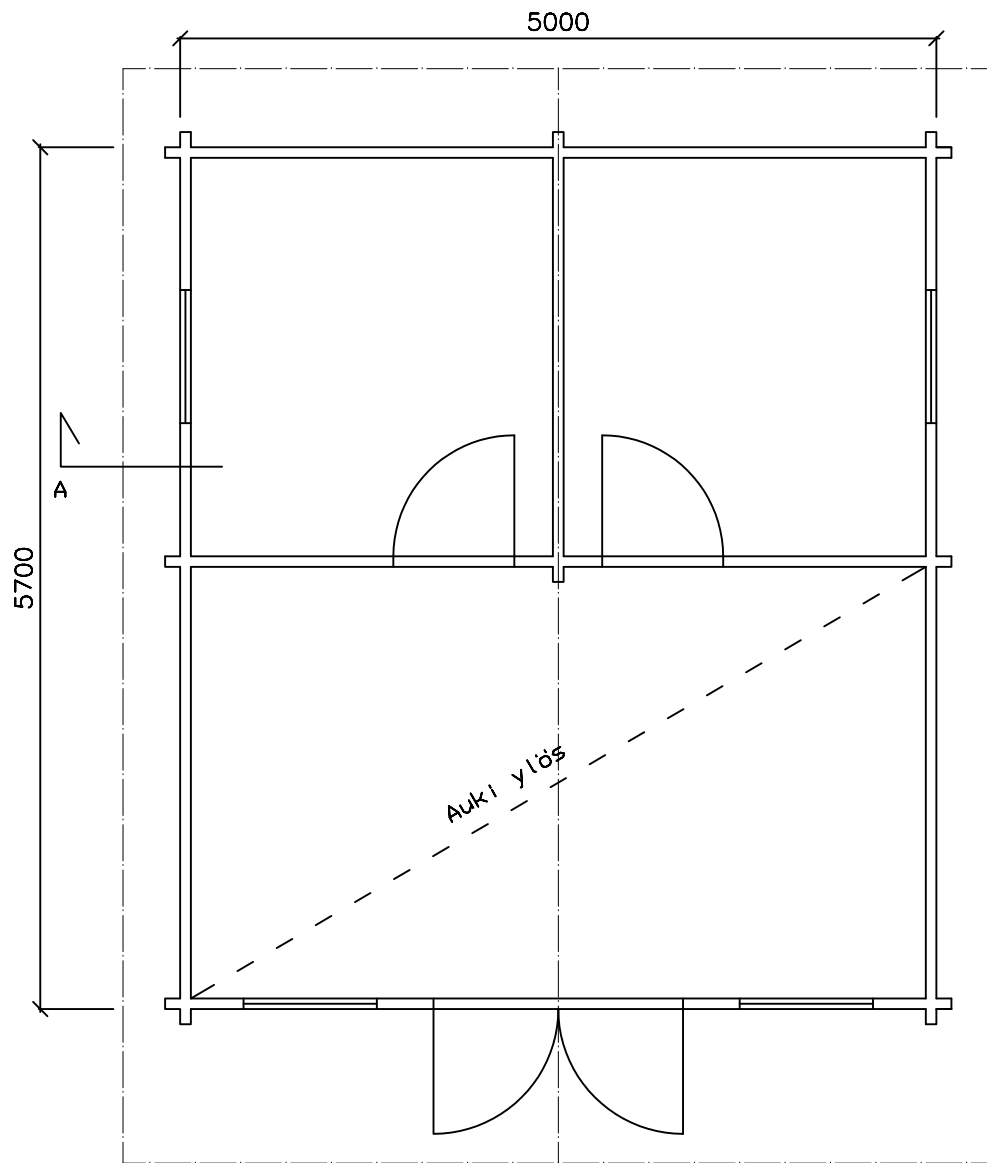
Pohjapiirros
