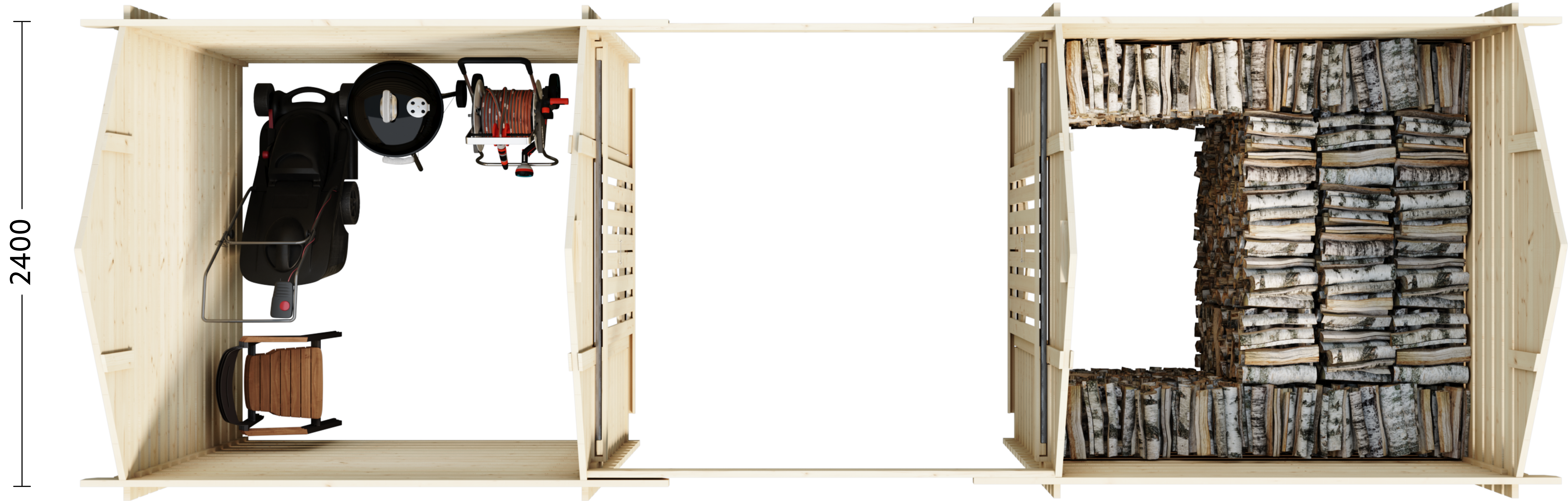
Huoneala / Room area 5,4 m 2 Katoksen ala / Canopy area 5,8 m 2 Huoneala / Room area 5,4 m 2
